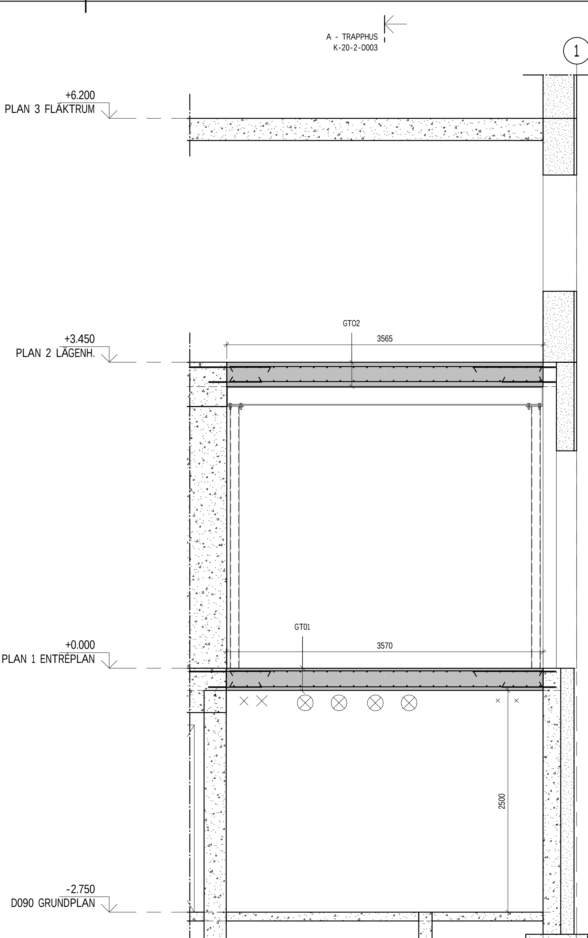
B-B 1 : 25
