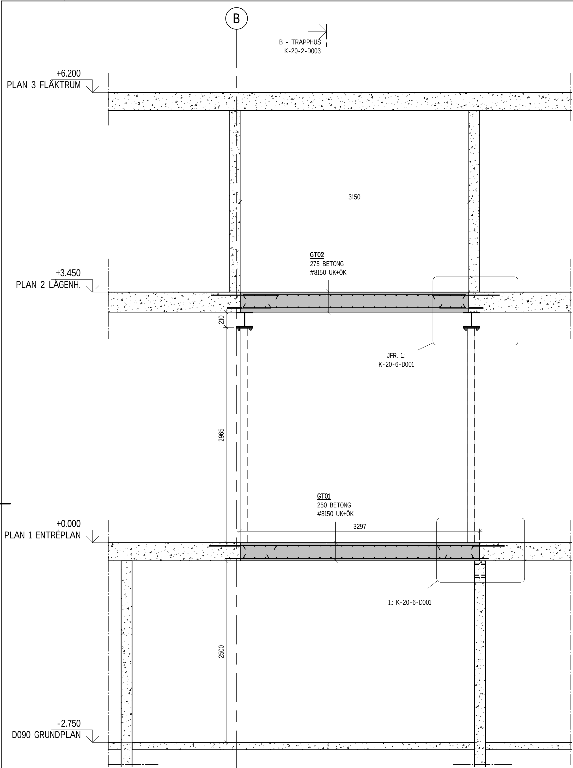
A-A 1 : 25
